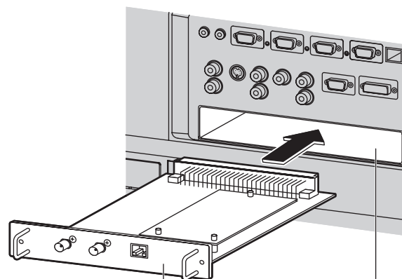
Slot
