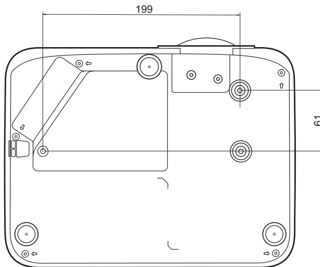
LS550W / LS550WH
